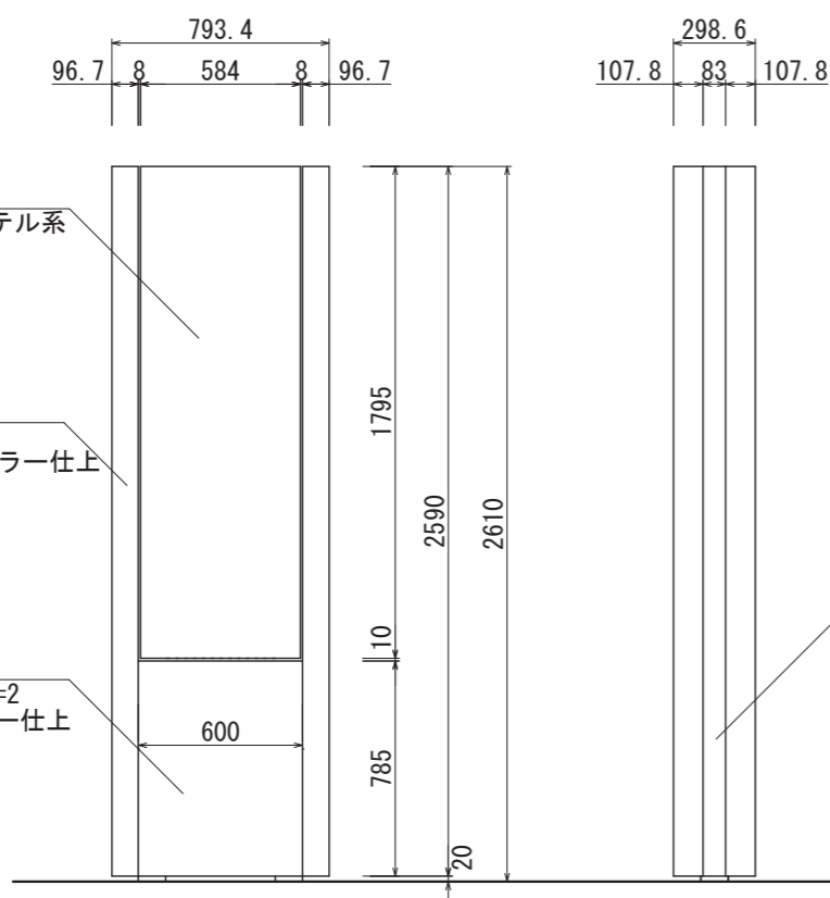
【正面図 S=1:30】
