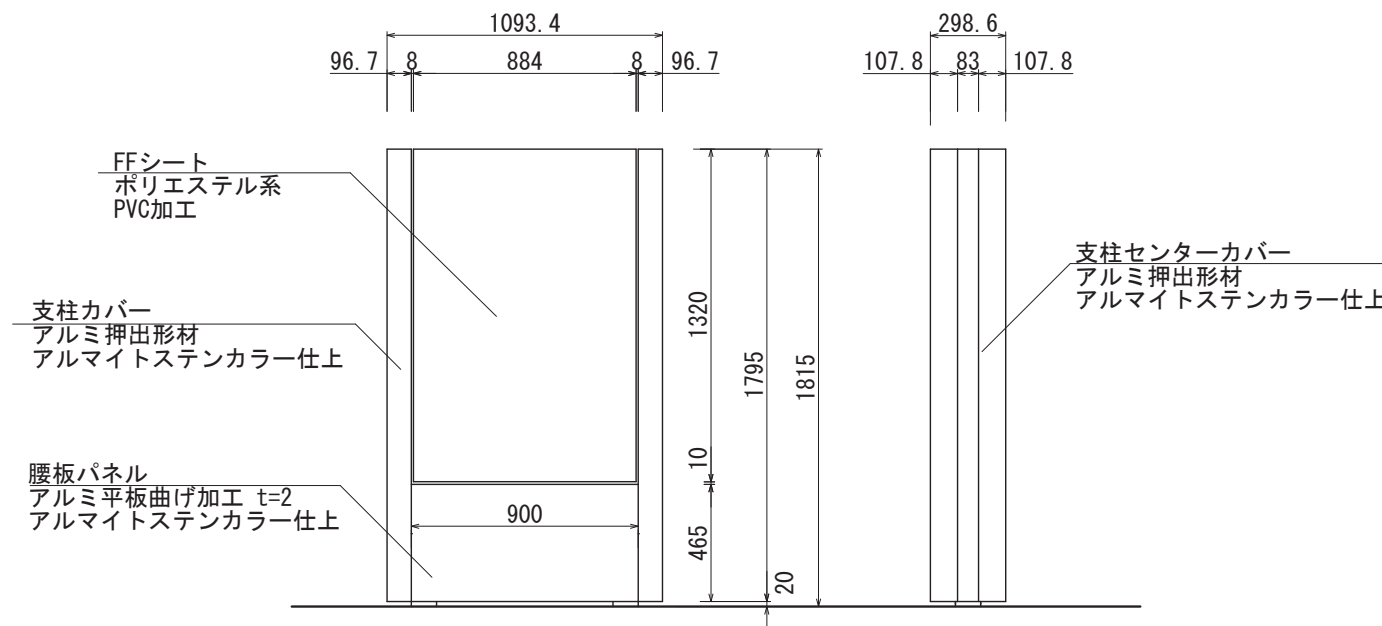
【正面図 S=1:30】
