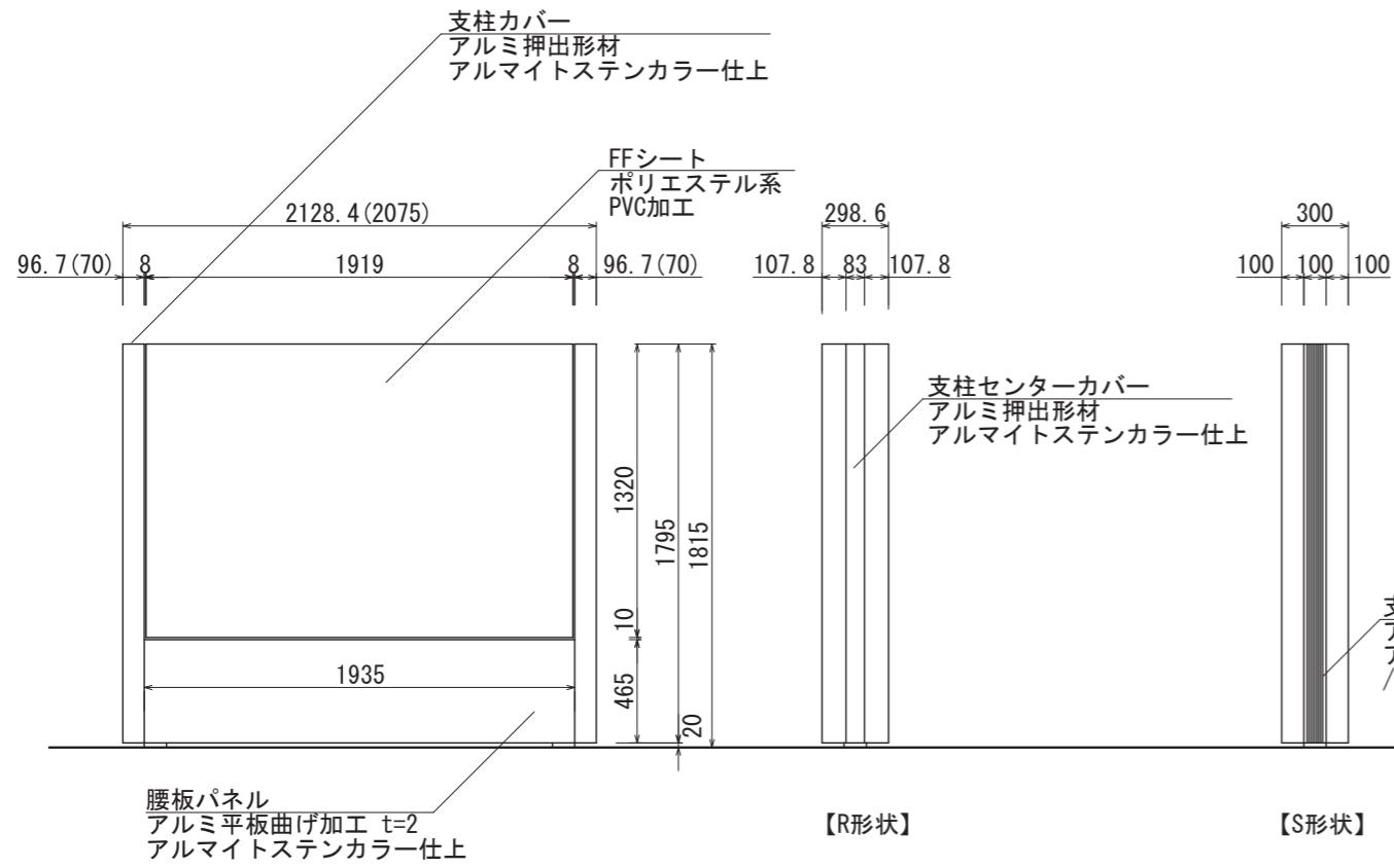
【看板本体正面図 S=1:35】
