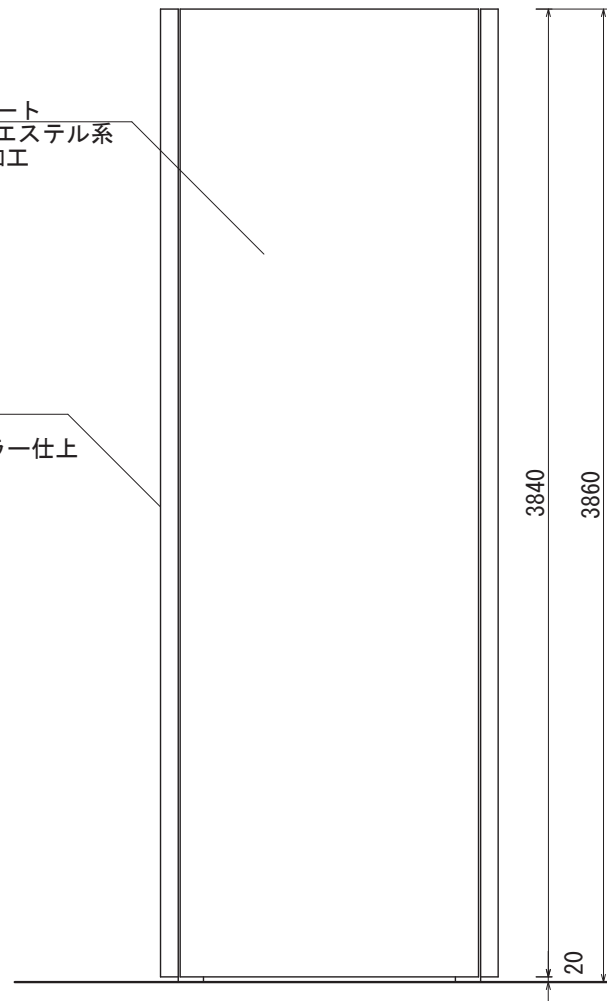
【正面図 S=1:30】
