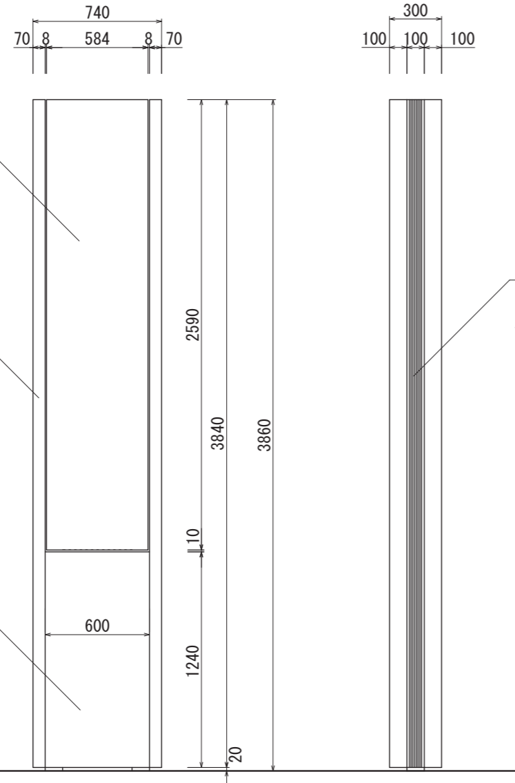
【正面図 S=1:30】
