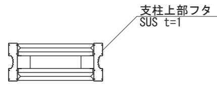
【平面図 S=1:30】
