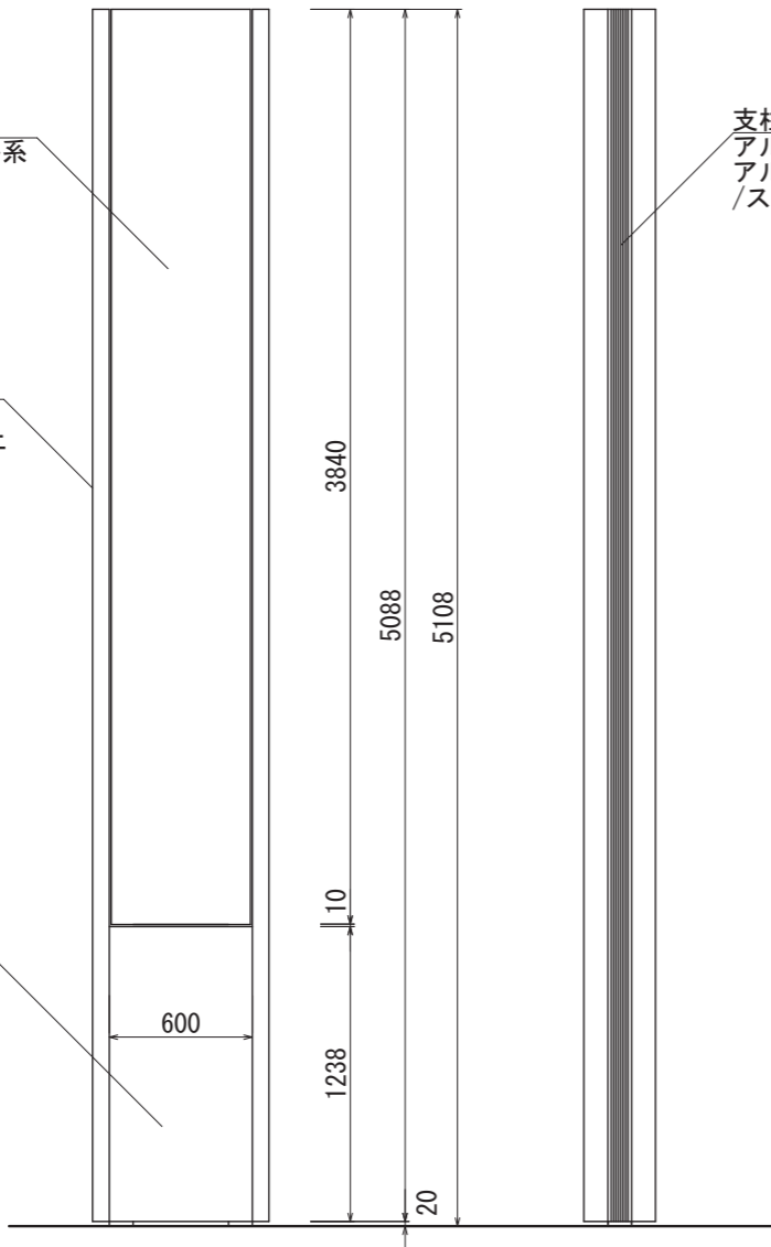
【正面図 S=1:35】
