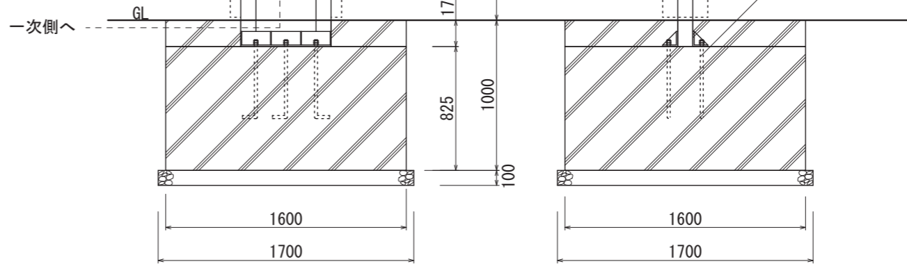
【鉄骨正面図 S=1:35】
