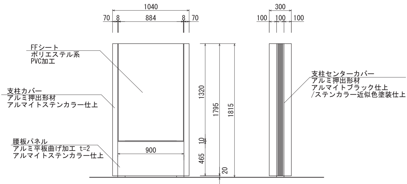
【正面図 S=1:30】
