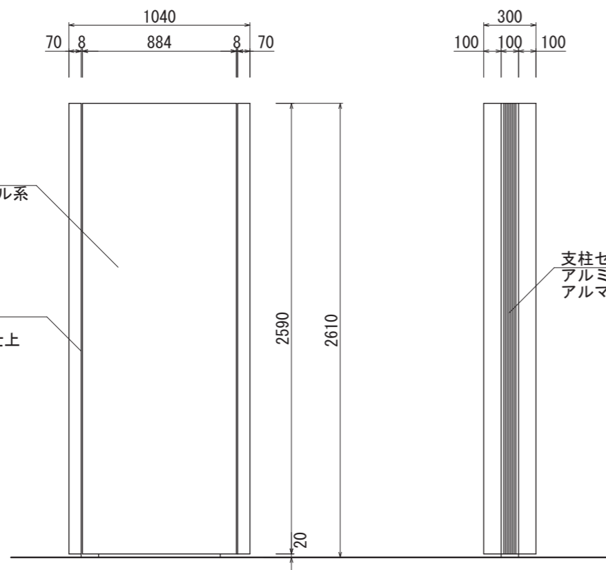
【正面図 S=1:30】
