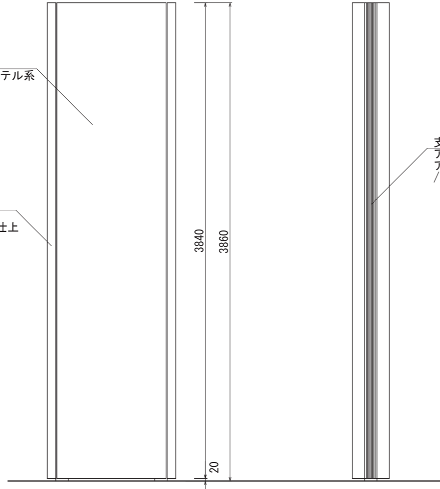
【正面図 S=1:30】
