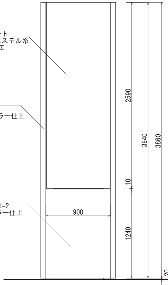
【正面図 S=1:30】
