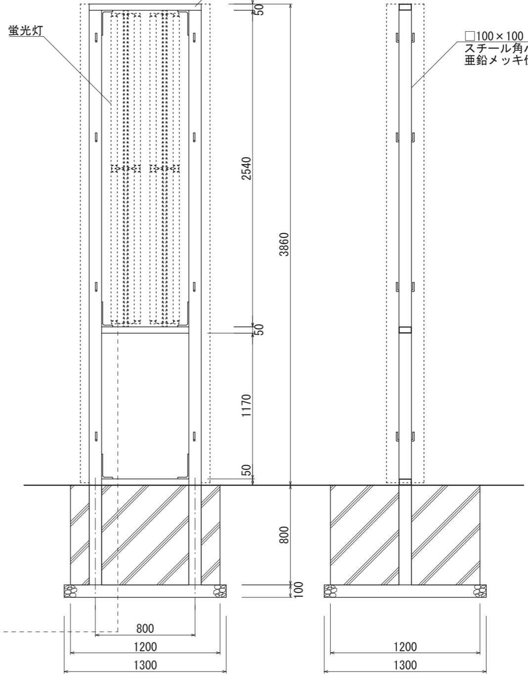
【鉄骨正面図 S=1:30】
