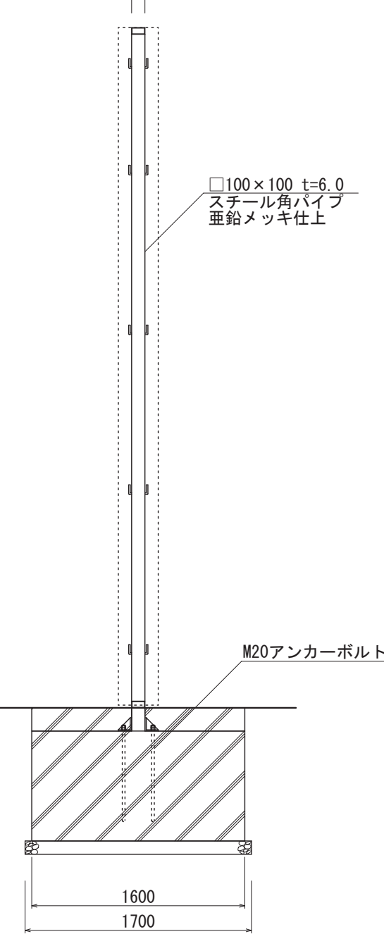
【鉄骨断面図 S=1:40】
