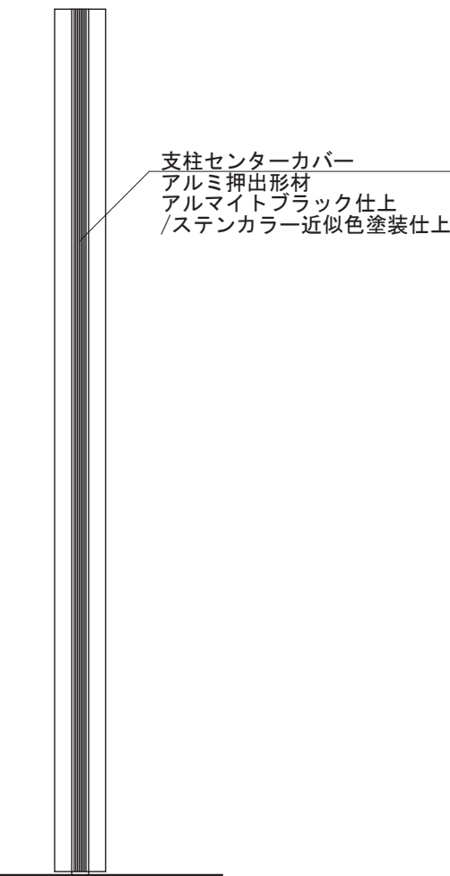
【側面図 S=1:40】
