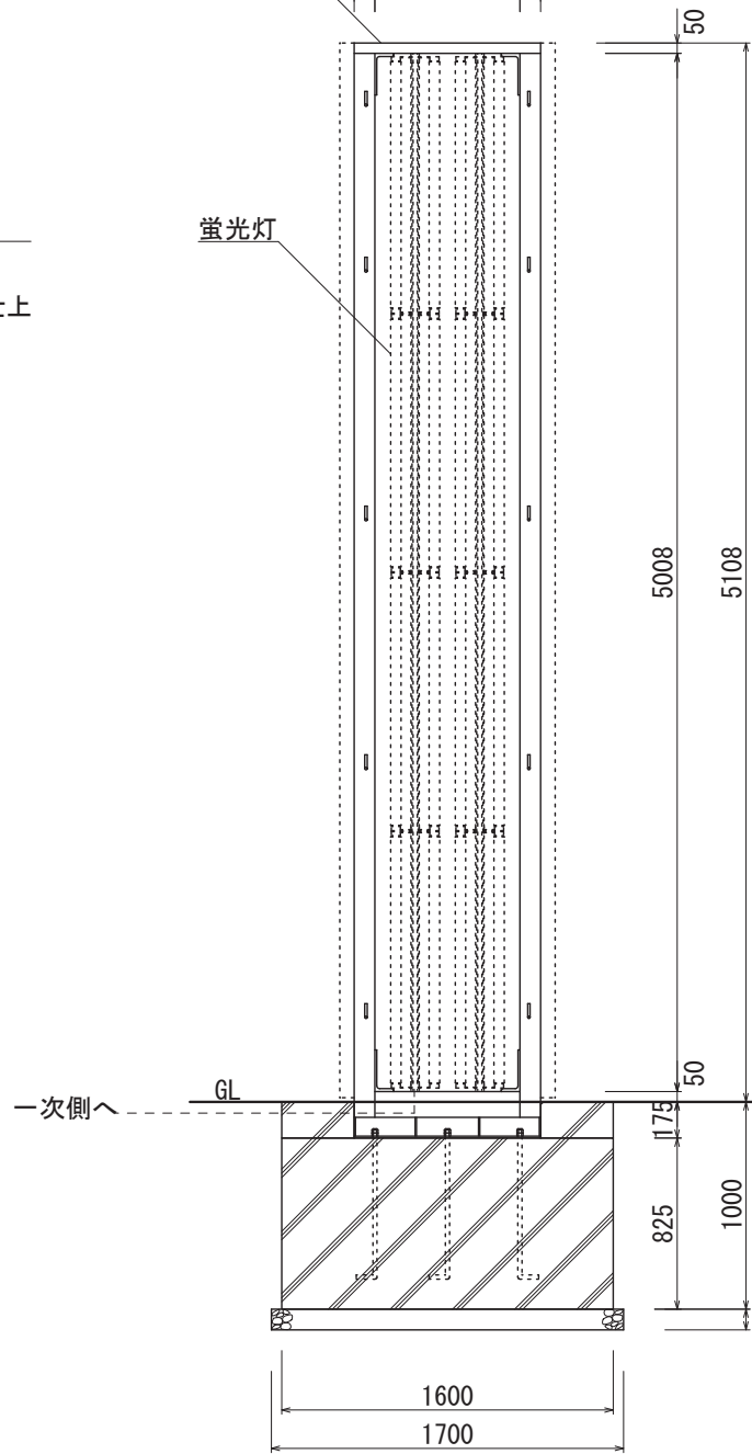
【鉄骨正面図 S=1:40】
