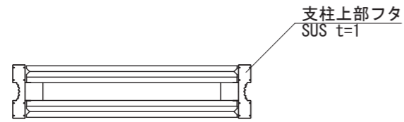
【平面図 S=1:30】
