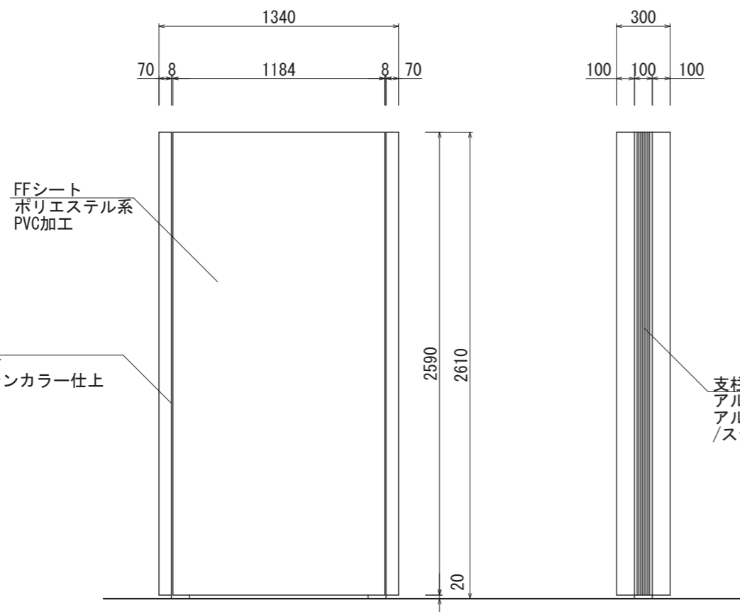
【正面図 S=1:30】
