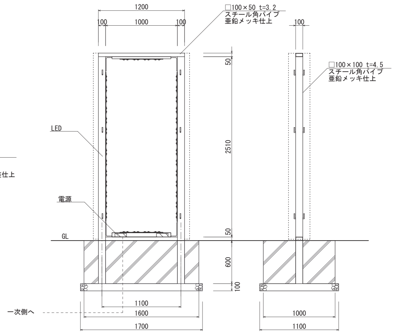
【鉄骨正面図 S=1:30】
