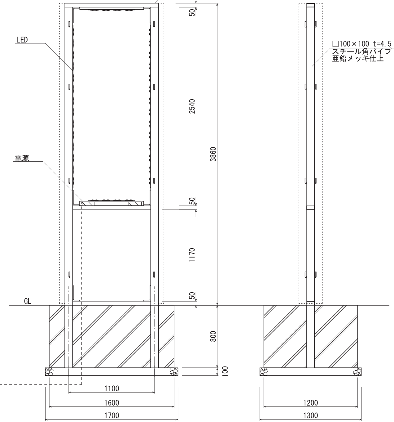
【鉄骨正面図 S=1:30】
