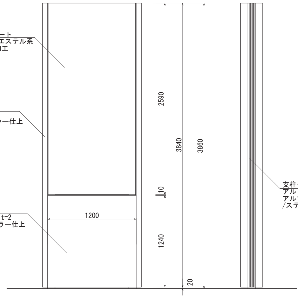
【正面図 S=1:30】
