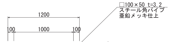
【断面図 S=1:30】
