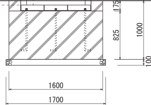
【鉄骨正面図 S=1:40】
