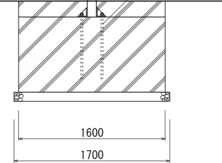
【鉄骨断面図 S=1:40】
