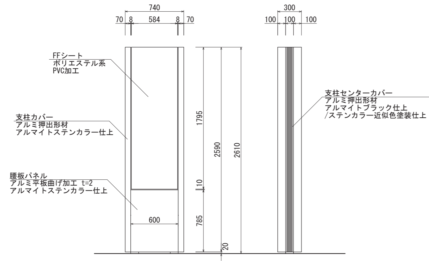
【正面図 S=1:30】
