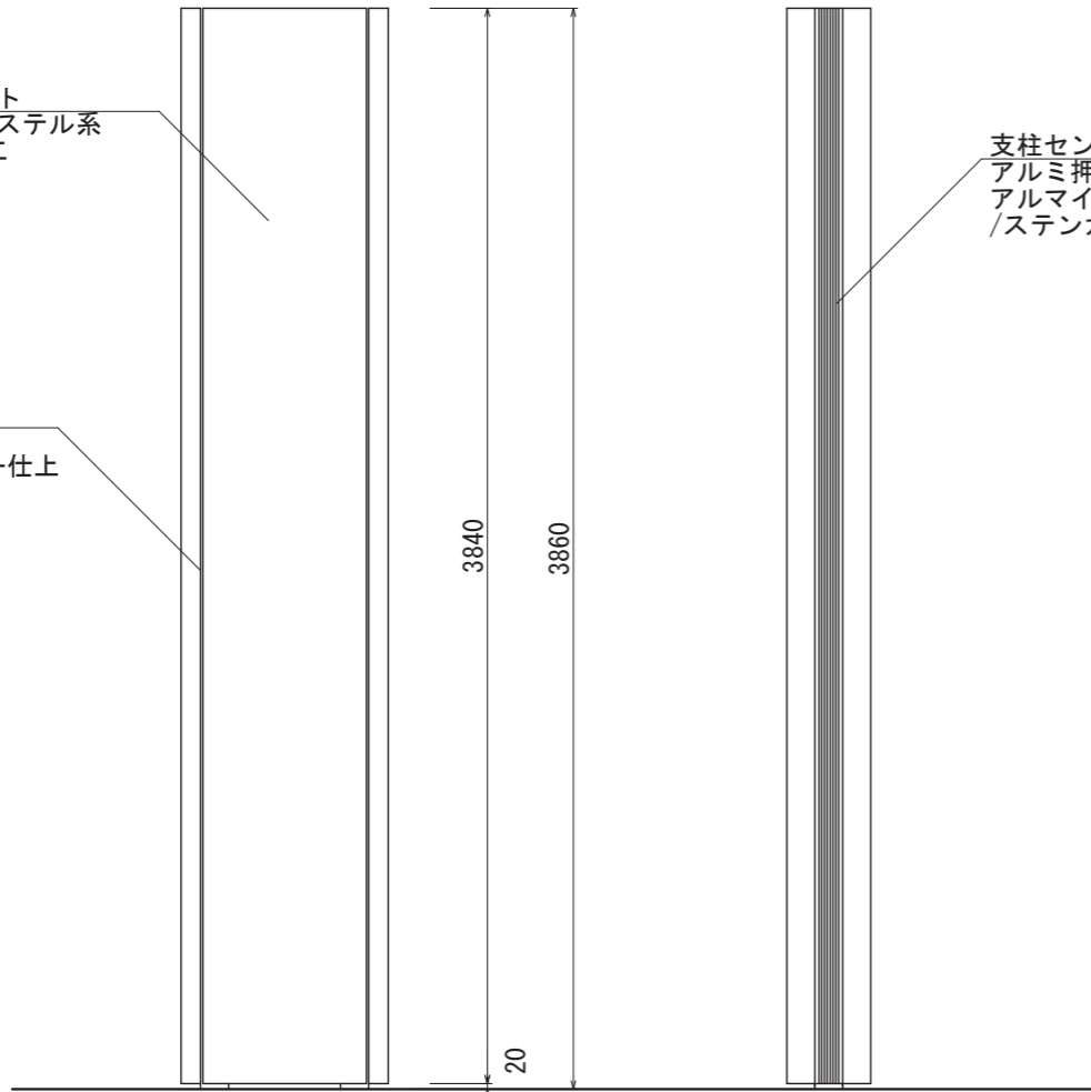
【正面図 S=1:30】
