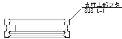
【平面図 S=1:30】
