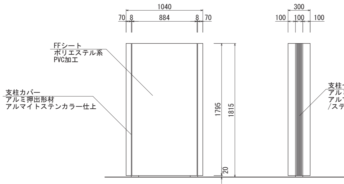
【正面図 S=1:30】
