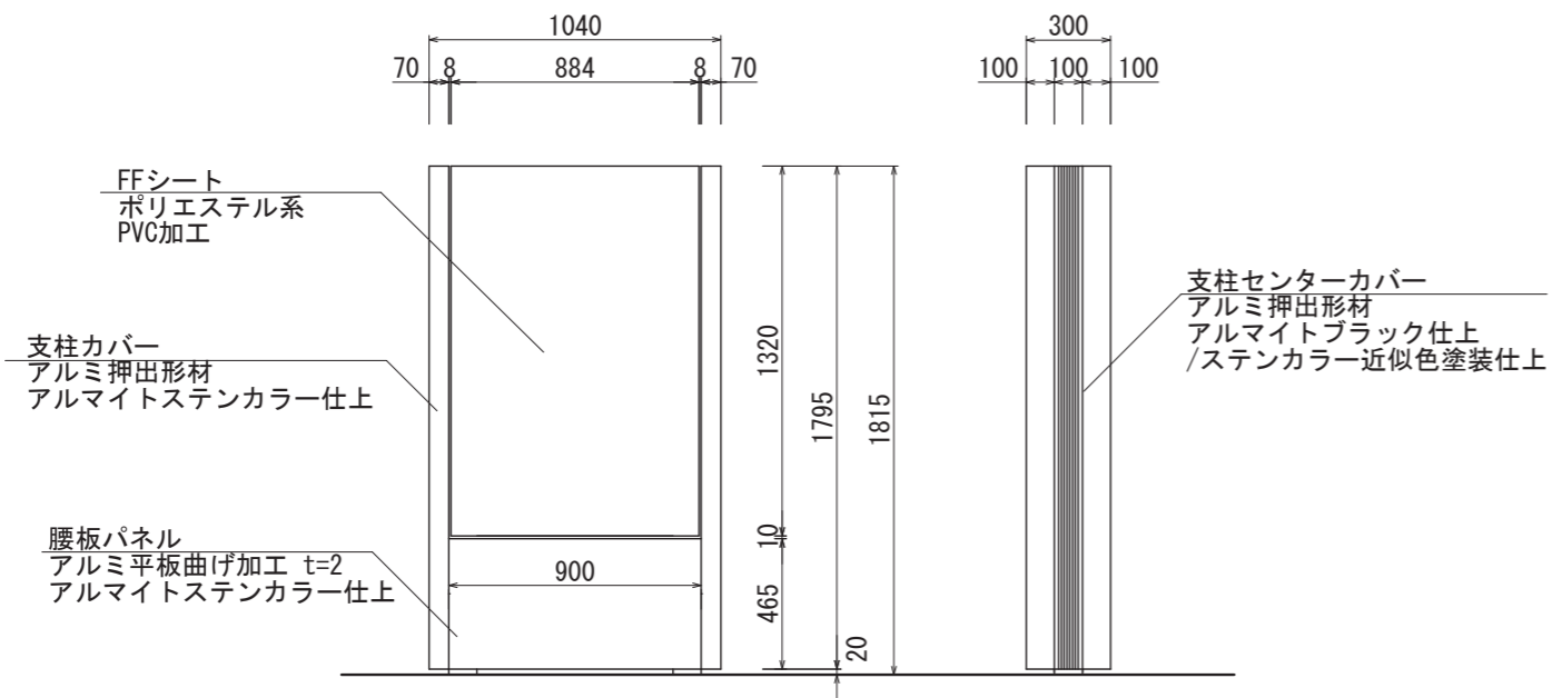
【正面図 S=1:30】
