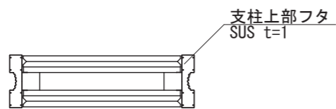
【平面図 S=1:30】
