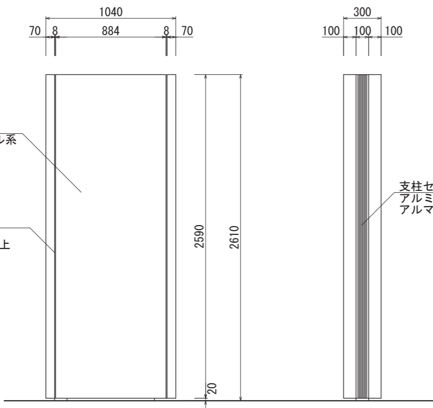
【正面図 S=1:30】
