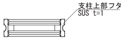
【平面図 S=1:40】
