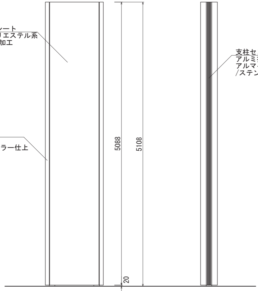
【正面図 S=1:40】
