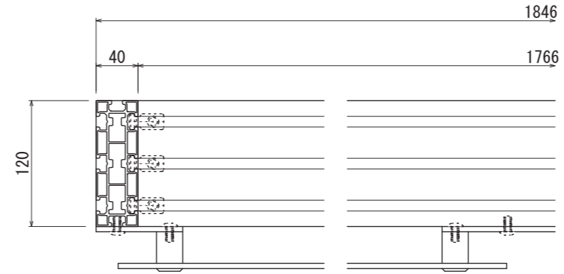
【平面図 S=1:5】
