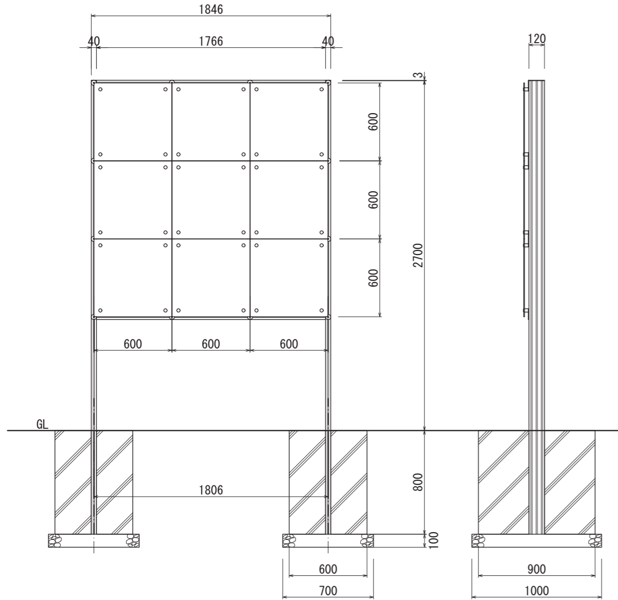
【正面図 S=1:30】
