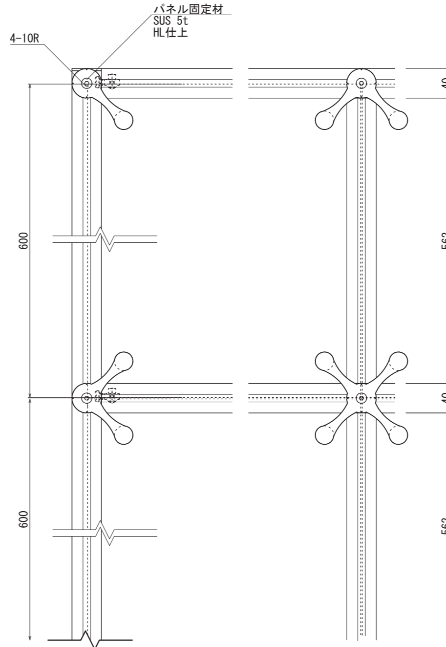
【正面図 S=1:5】
