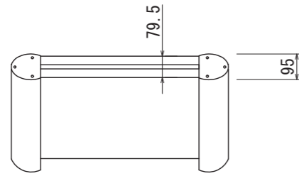
【平面図 S=1:20】
