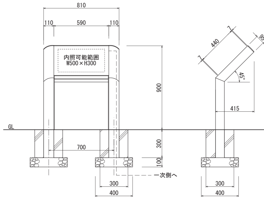
【側面図 S=1:20】
