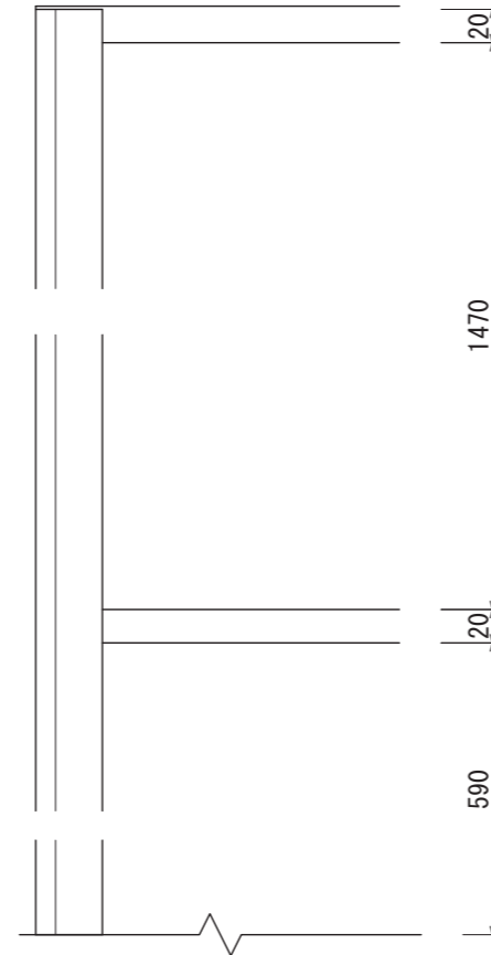
【正面図 S=1:5】
