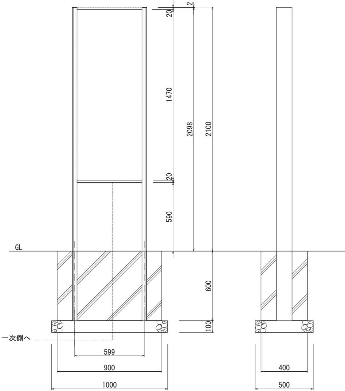
【正面図 S=1:20】
