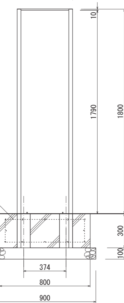
【側面図 S=1:20】
