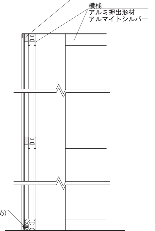
【断面図 S=1:5】
