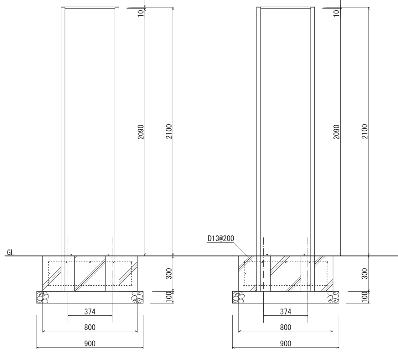
【正面図 S=1:20】
