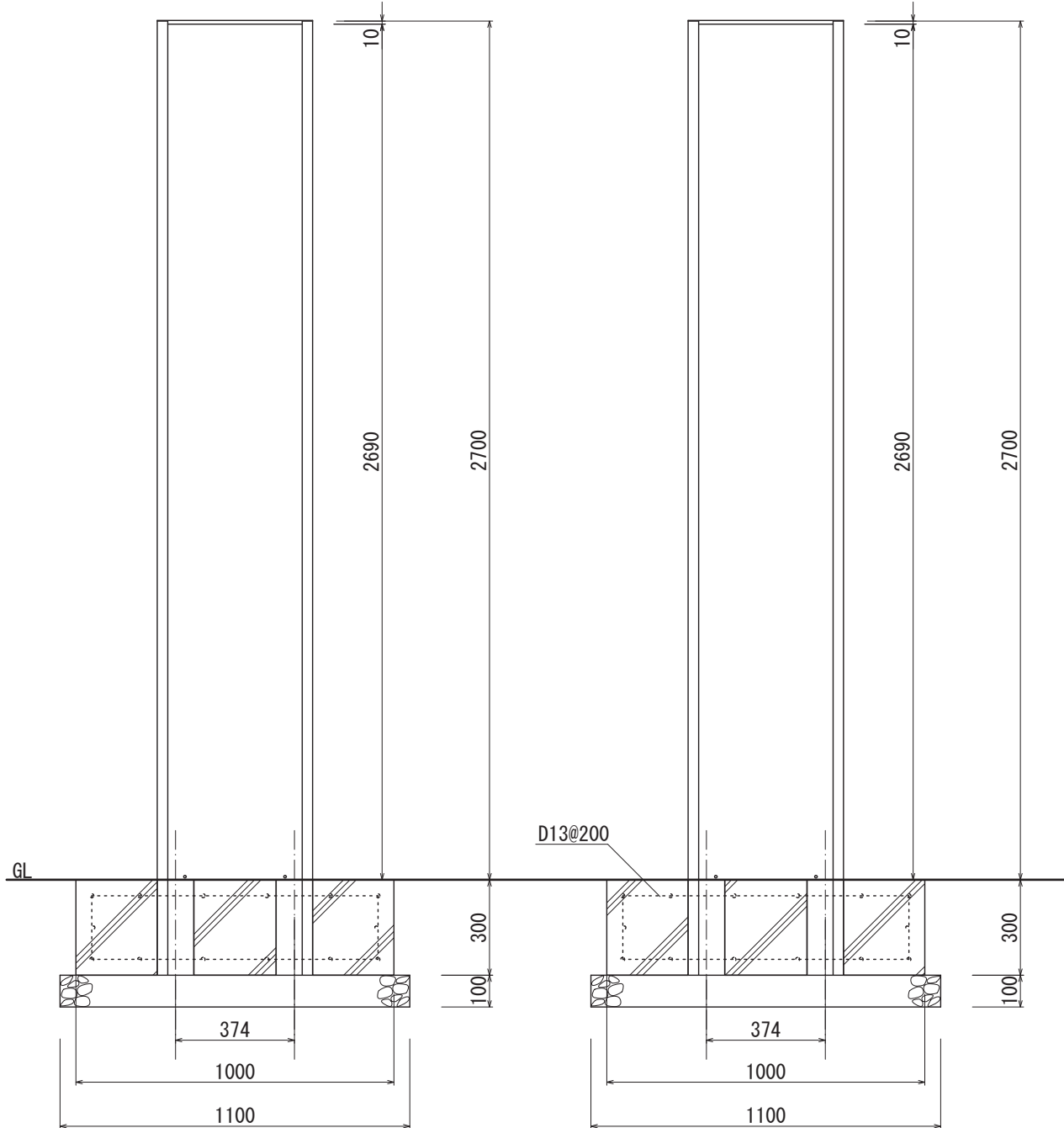
【正面図 S=1:20】
