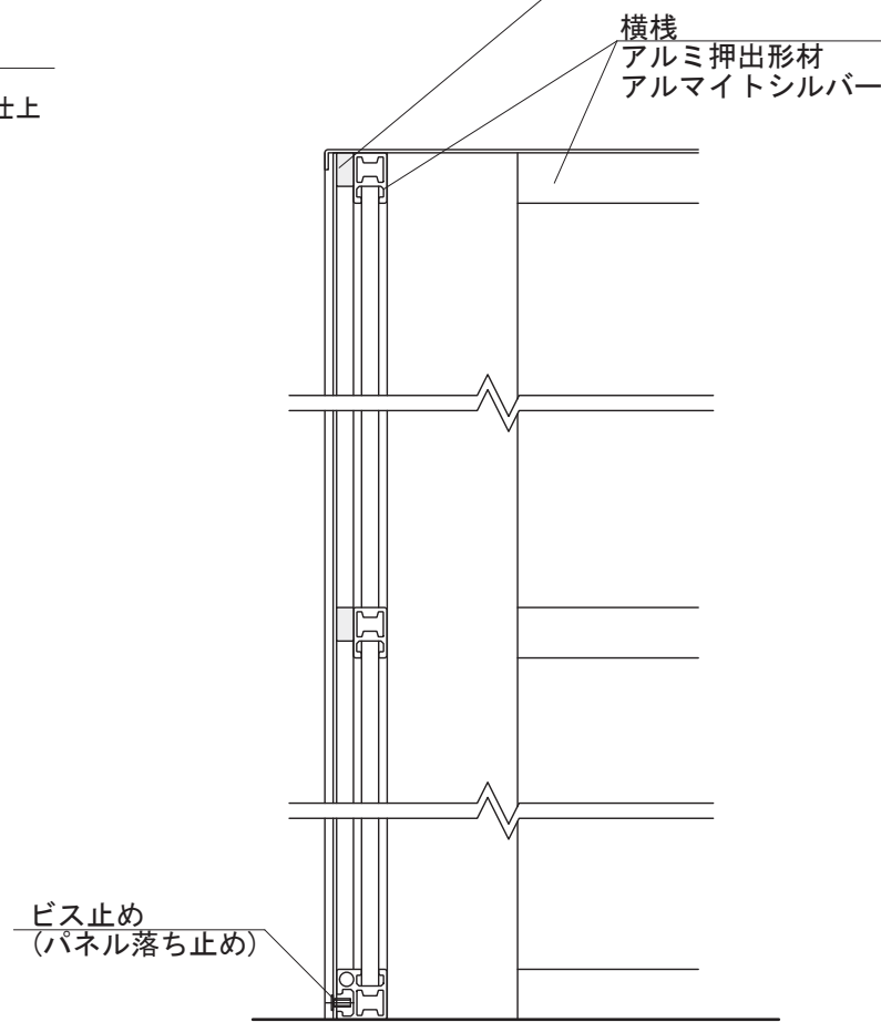
【断面図 S=1:5】
