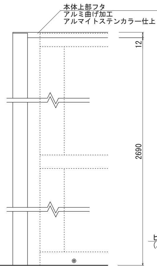
【正面図 S=1:5】
