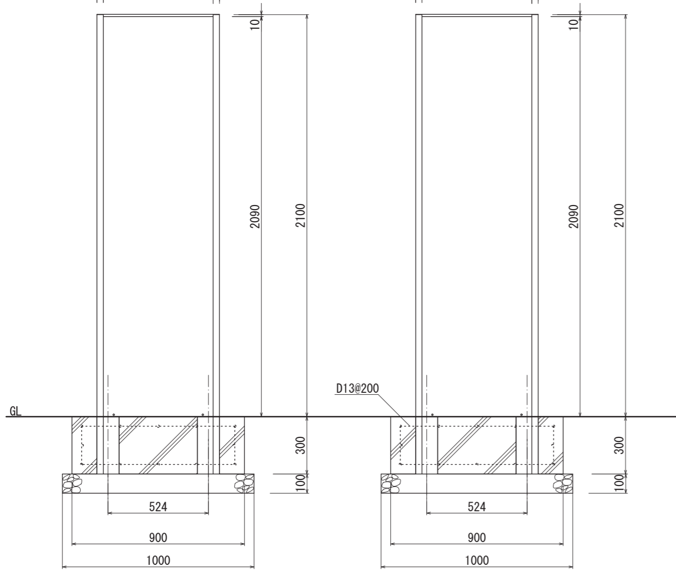
【正面図 S=1:20】
