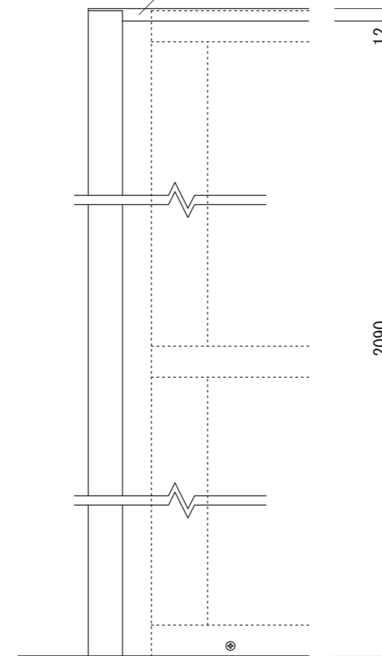
【正面図 S=1:5】
