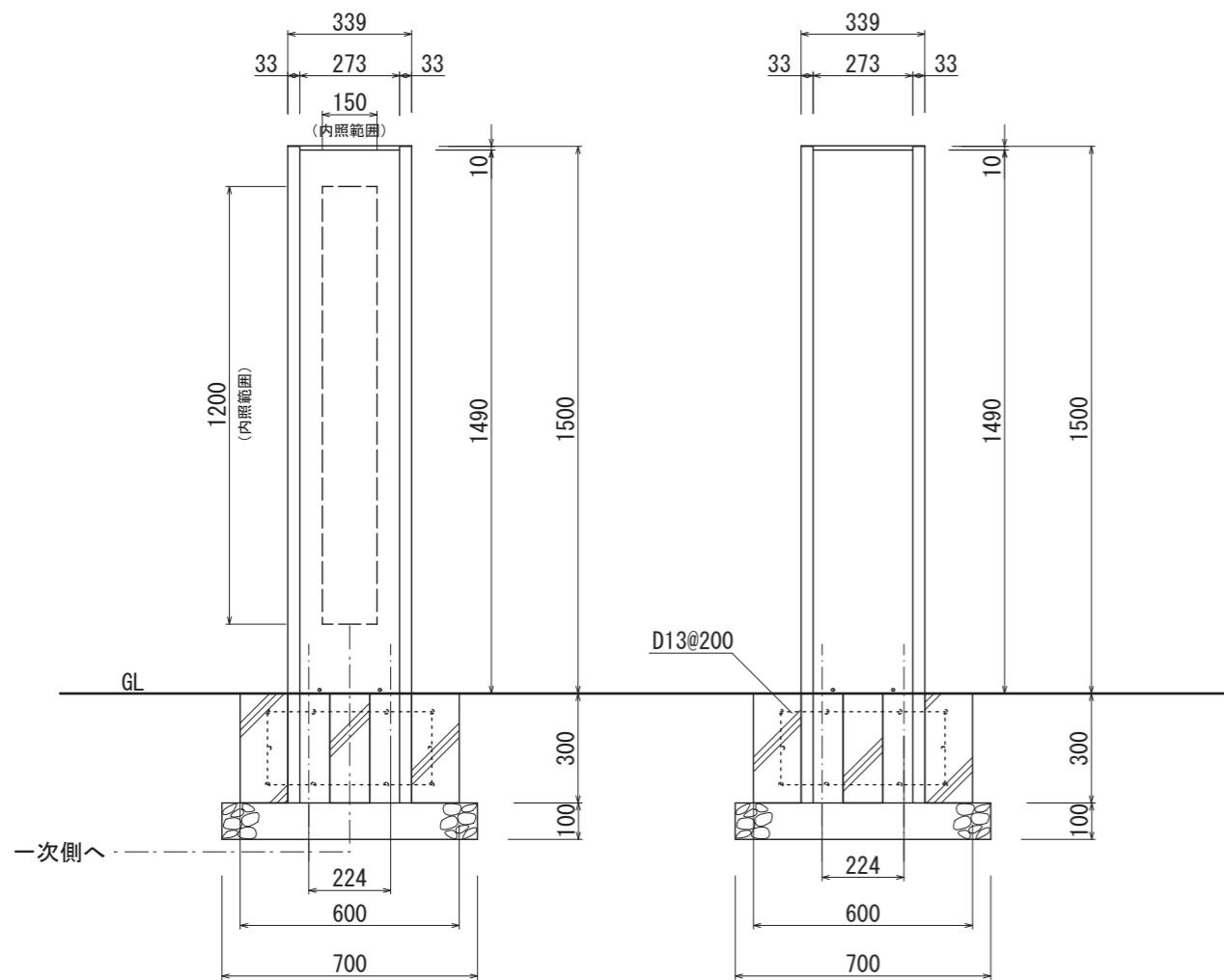
【正面図 S=1:20】
