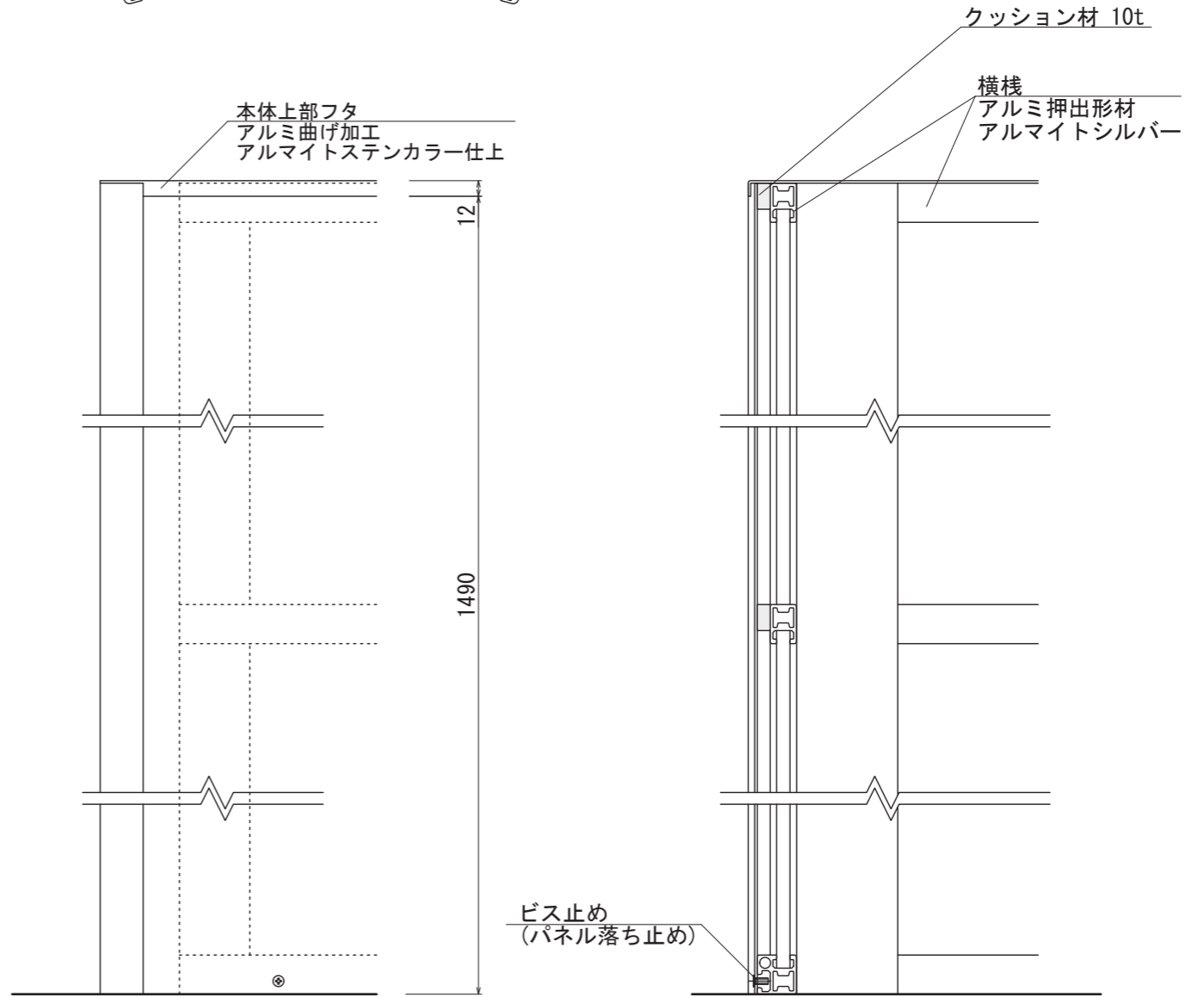
【正面図 S=1:5】
