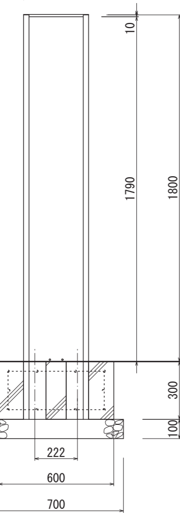
【正面図 S=1:20】
