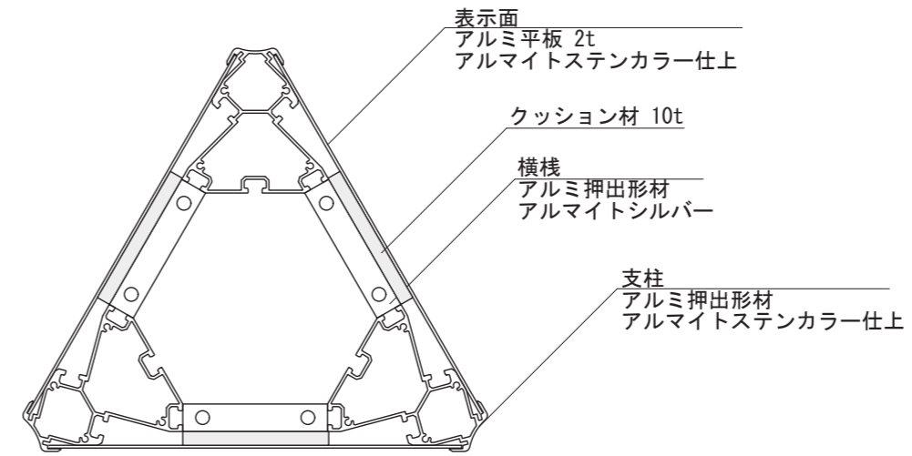
【断面図 S=1:5】
