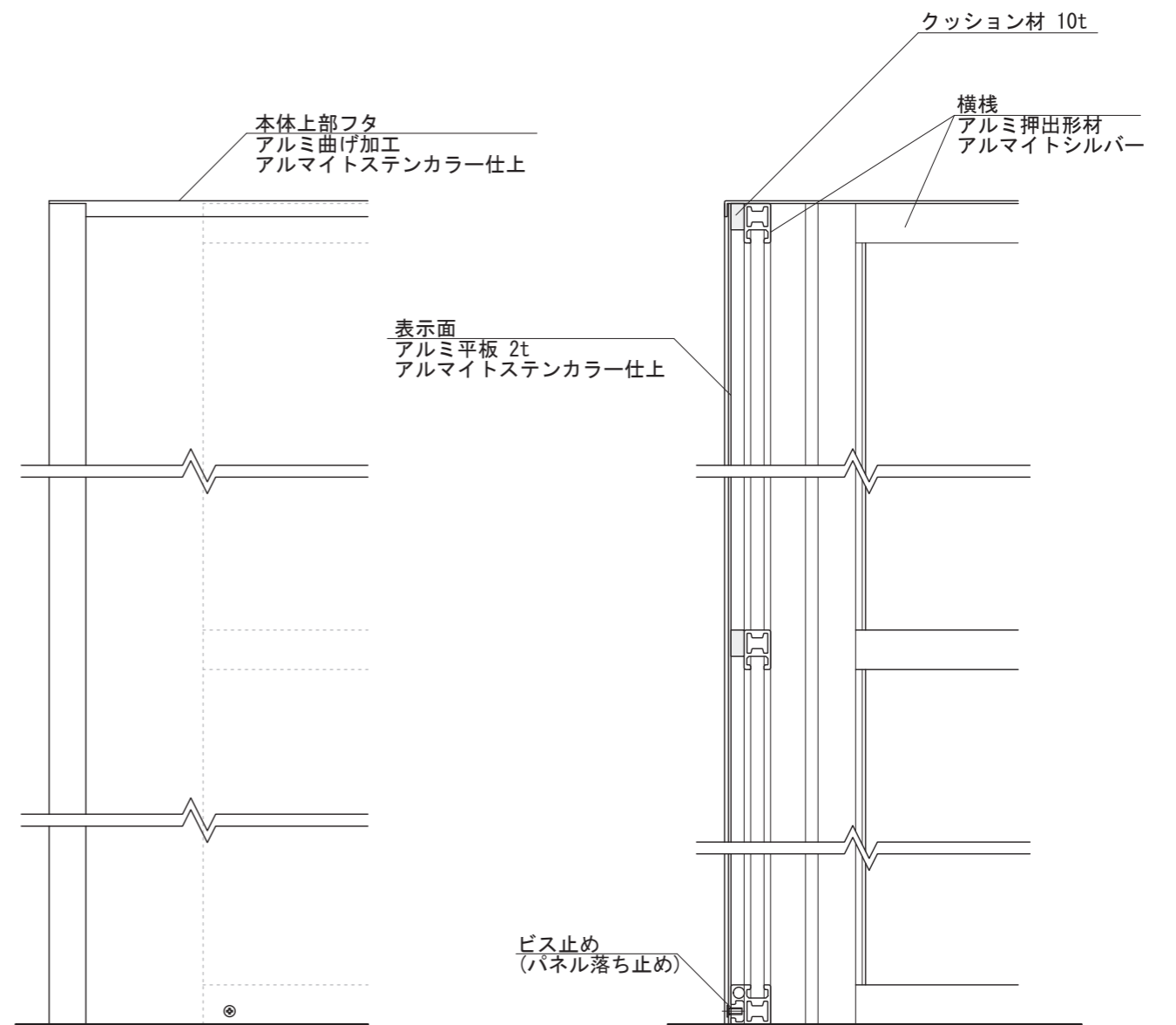
【断面図 S=1:5】
