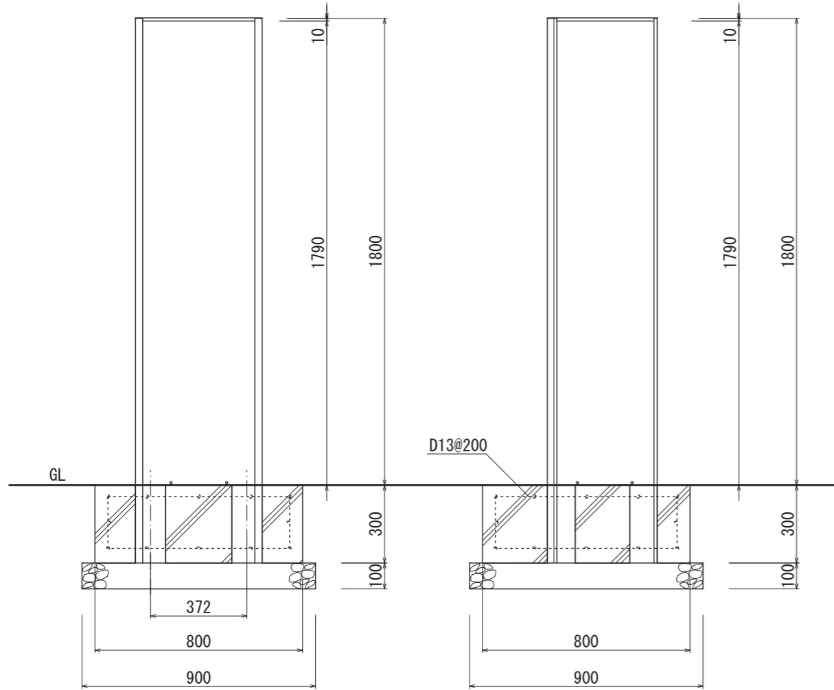
【正面図 S=1:20】
