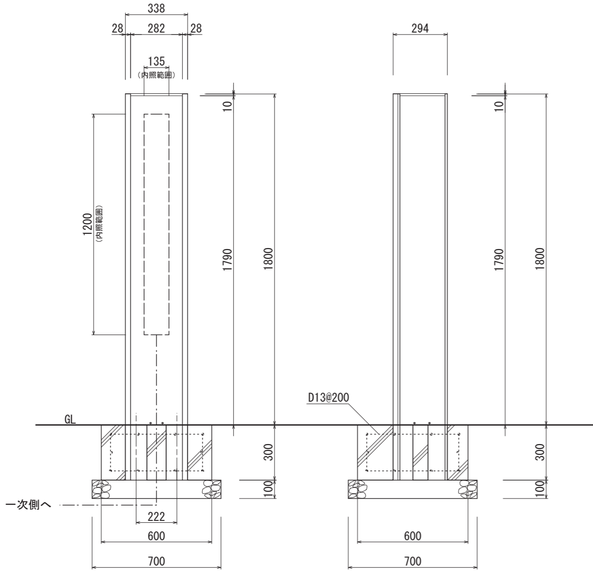
【正面図 S=1:20】
