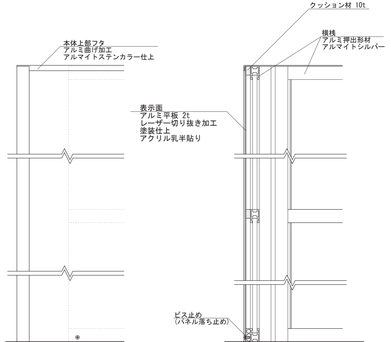
【正面図 S=1:5】
