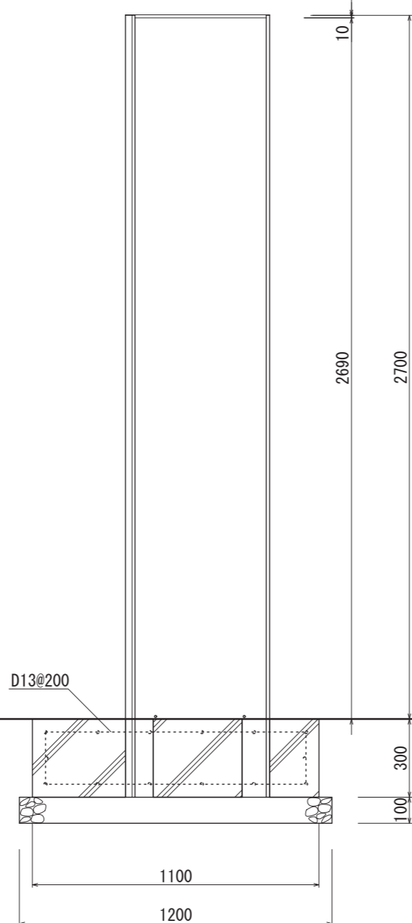
【側面図 S=1:20】
