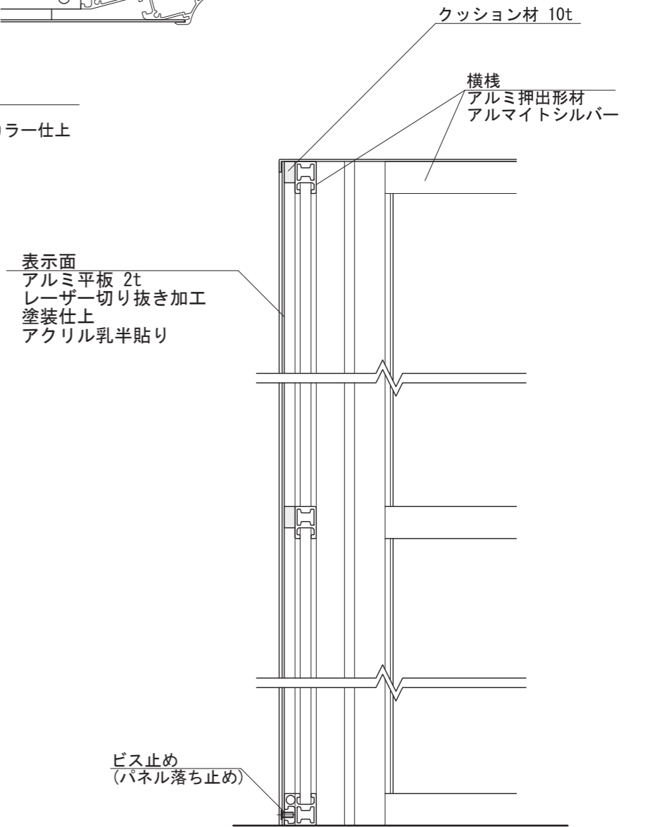
【断面図 S=1:5】
