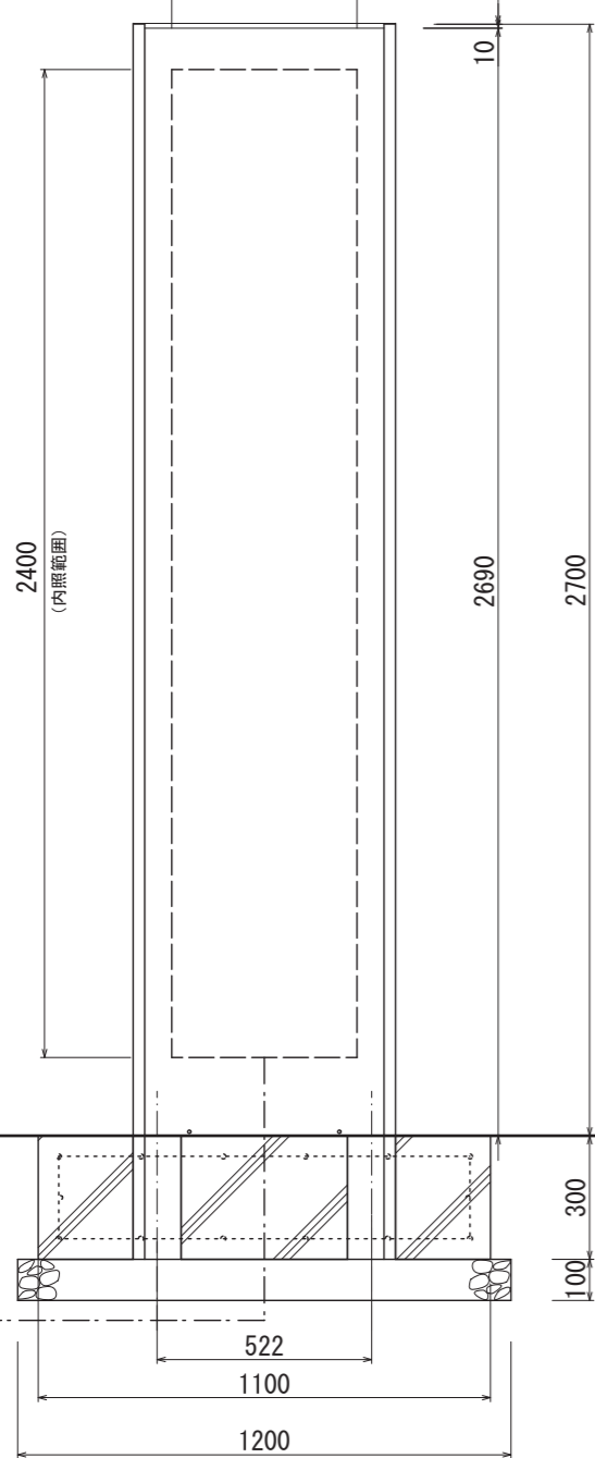
【正面図 S=1:20】
