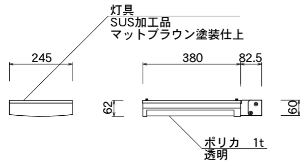
【灯具詳細図 1:15】
