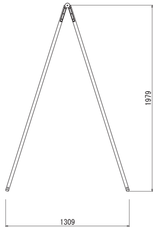
【側面図 S=1:25】
