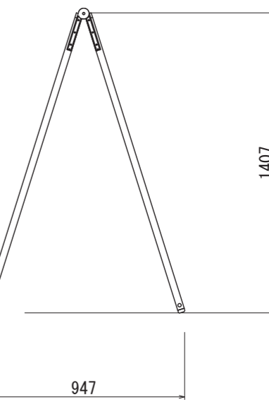
【側面図 S=1:25】
