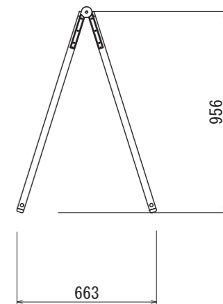
【側面図 S=1:25】
