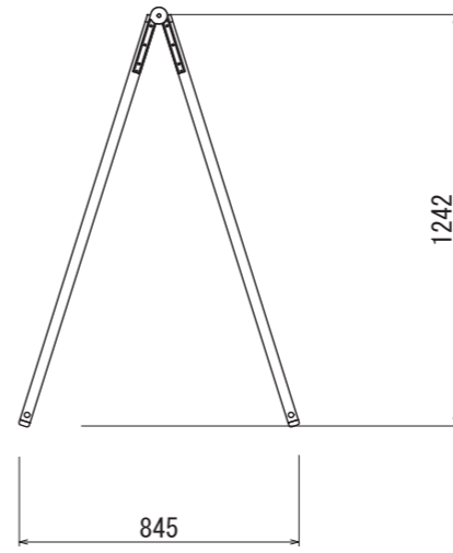
【側面図 S=1:25】
