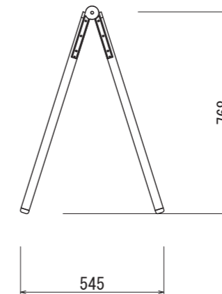
【側面図 S=1:20】
