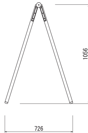
【側面図 S=1:20】
