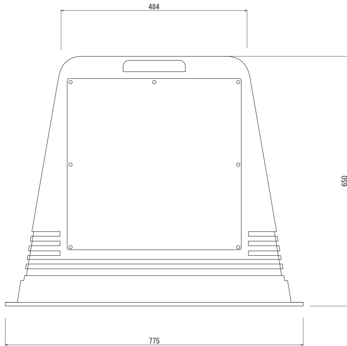
【正面図 S=1:6】
