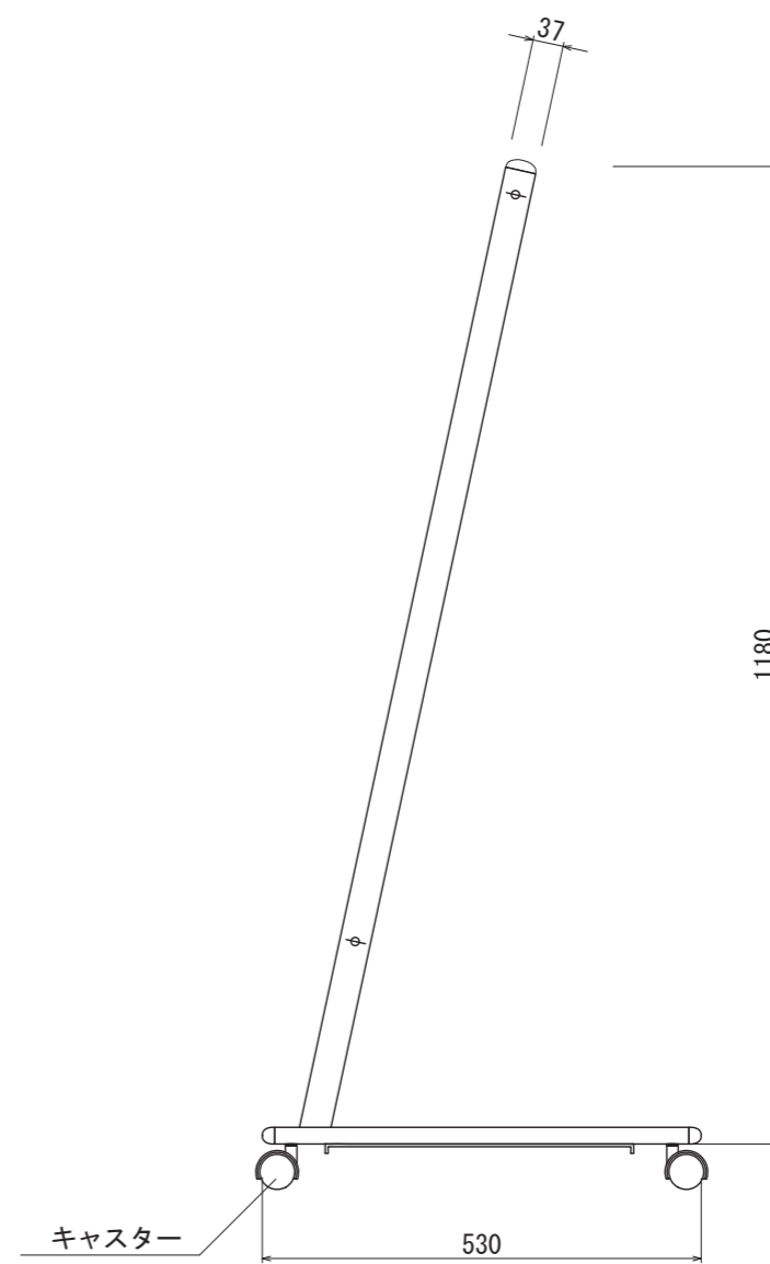
【側面図 S=1:10】
