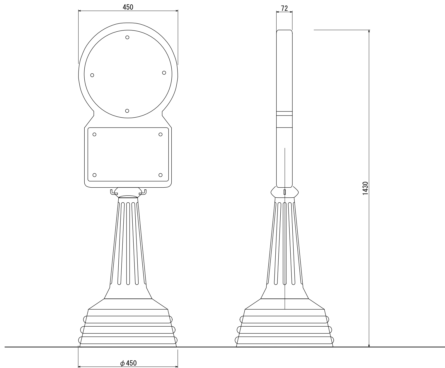
パークサインBタイプ
