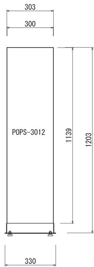
【正面図 S=1:15】
