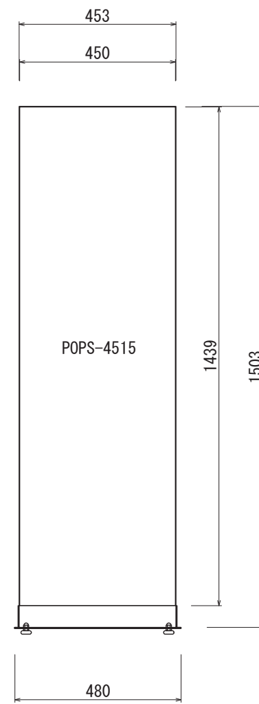
【正面図 S=1:15】
