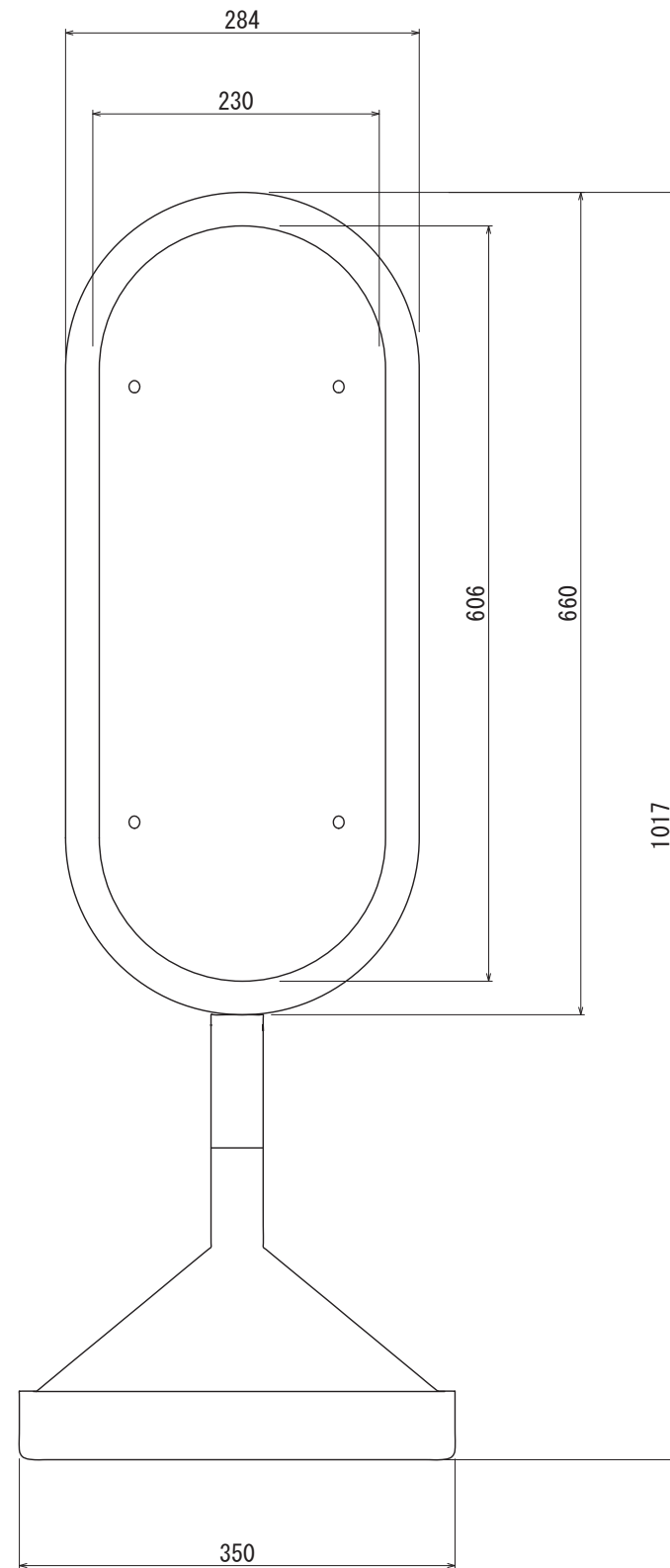
【正面図 S=1:6】
