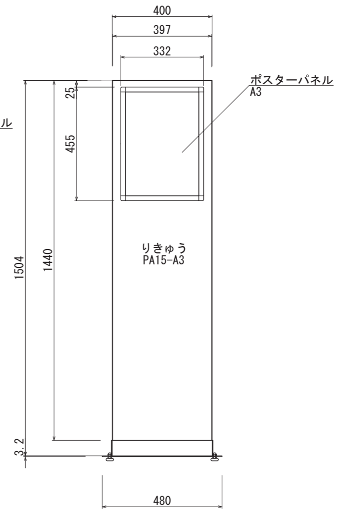
【正面図 S=1:15】
