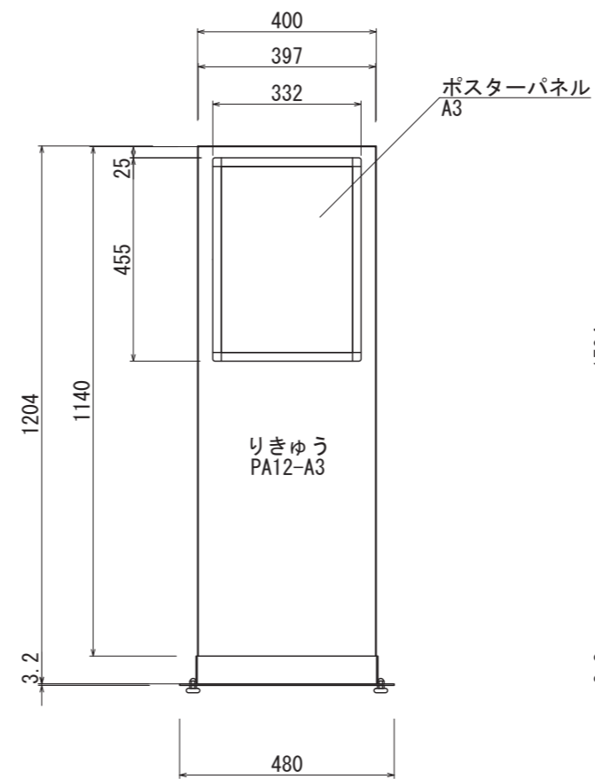
【正面図 S=1:15】
