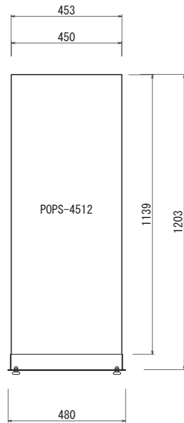
【正面図 S=1:15】
