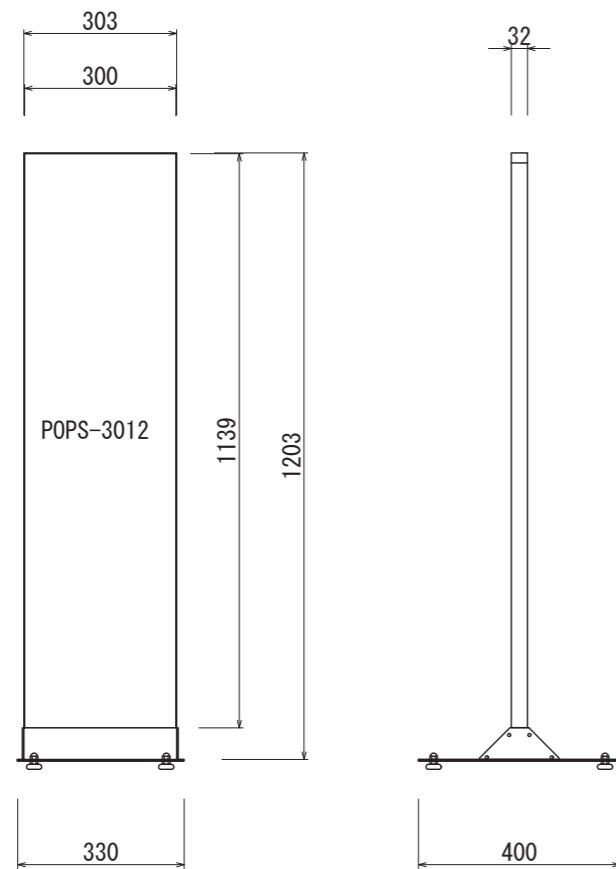
【正面図 S=1:15】
