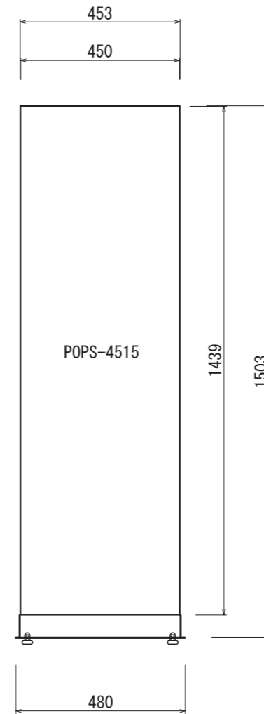
【正面図 S=1:15】
