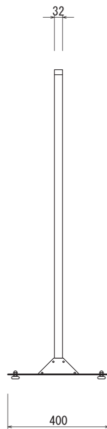
【側面図 S=1:15】
