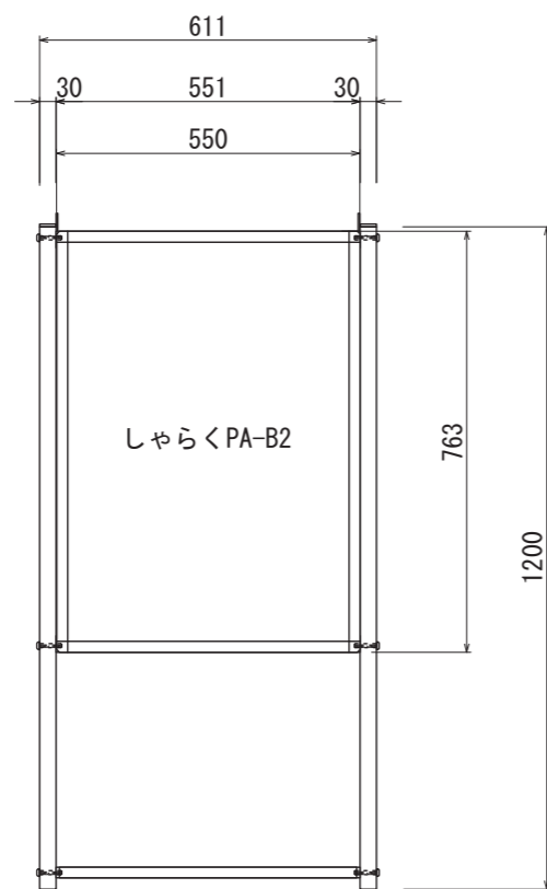
【正面図 S=1:15】
