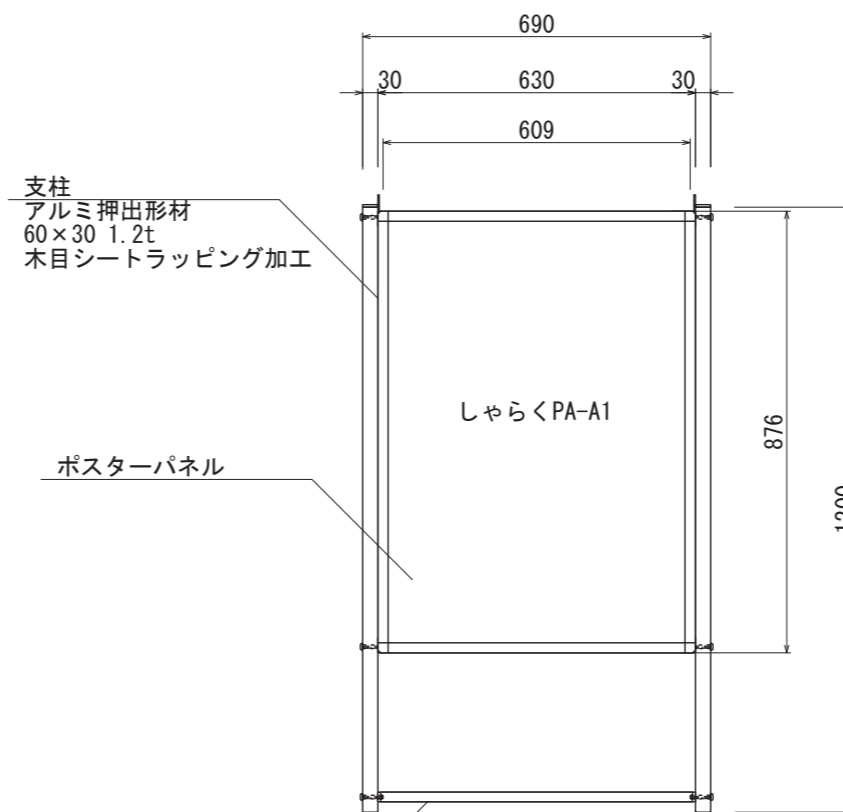
【正面図 S=1:15】
