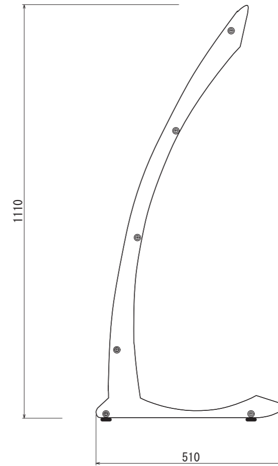
【側面図 S=1:10】
