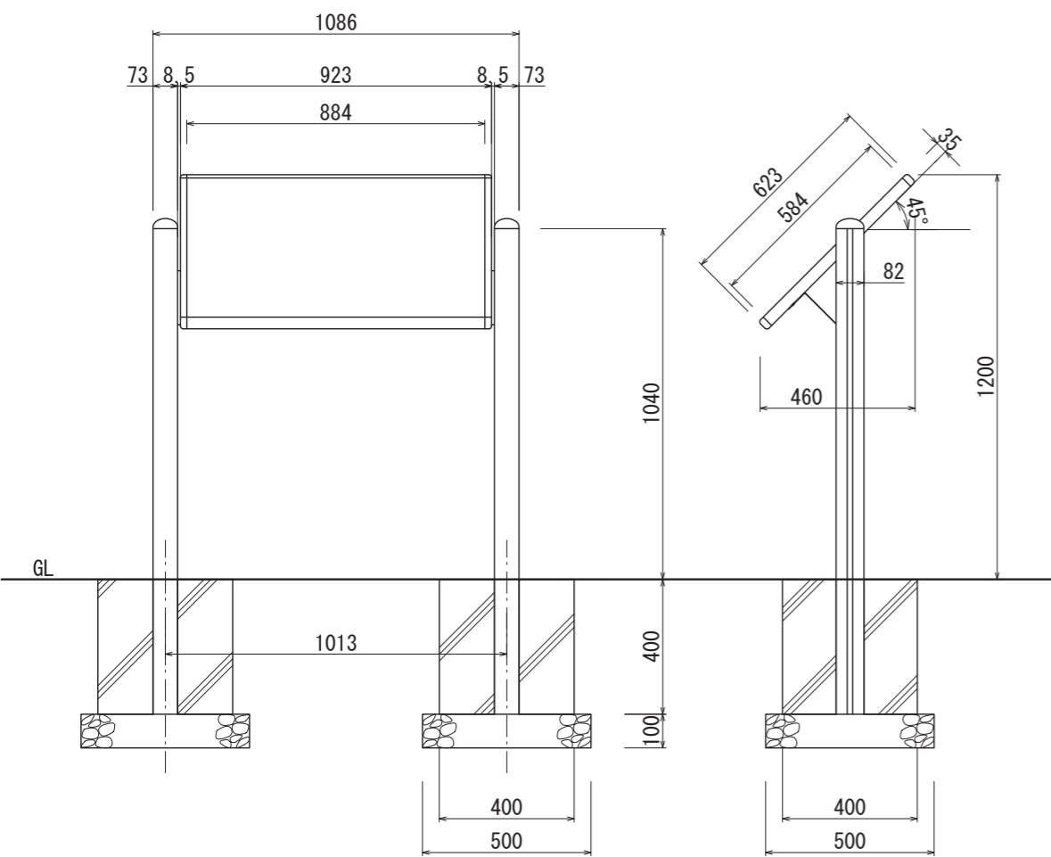
【正面図 S=1:20】
