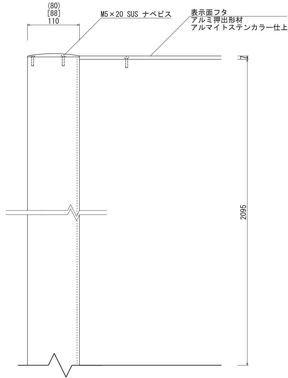
【正面図 S=1:5】
