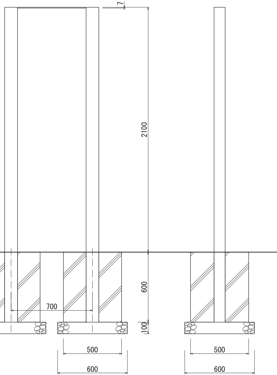
【正面図 S=1:20】
