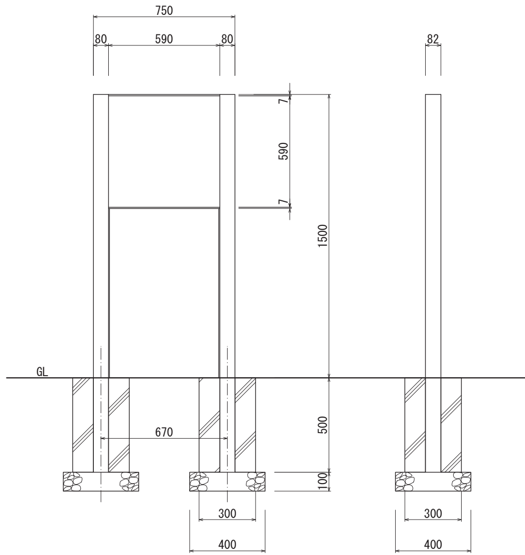
【正面図 S=1:20】
