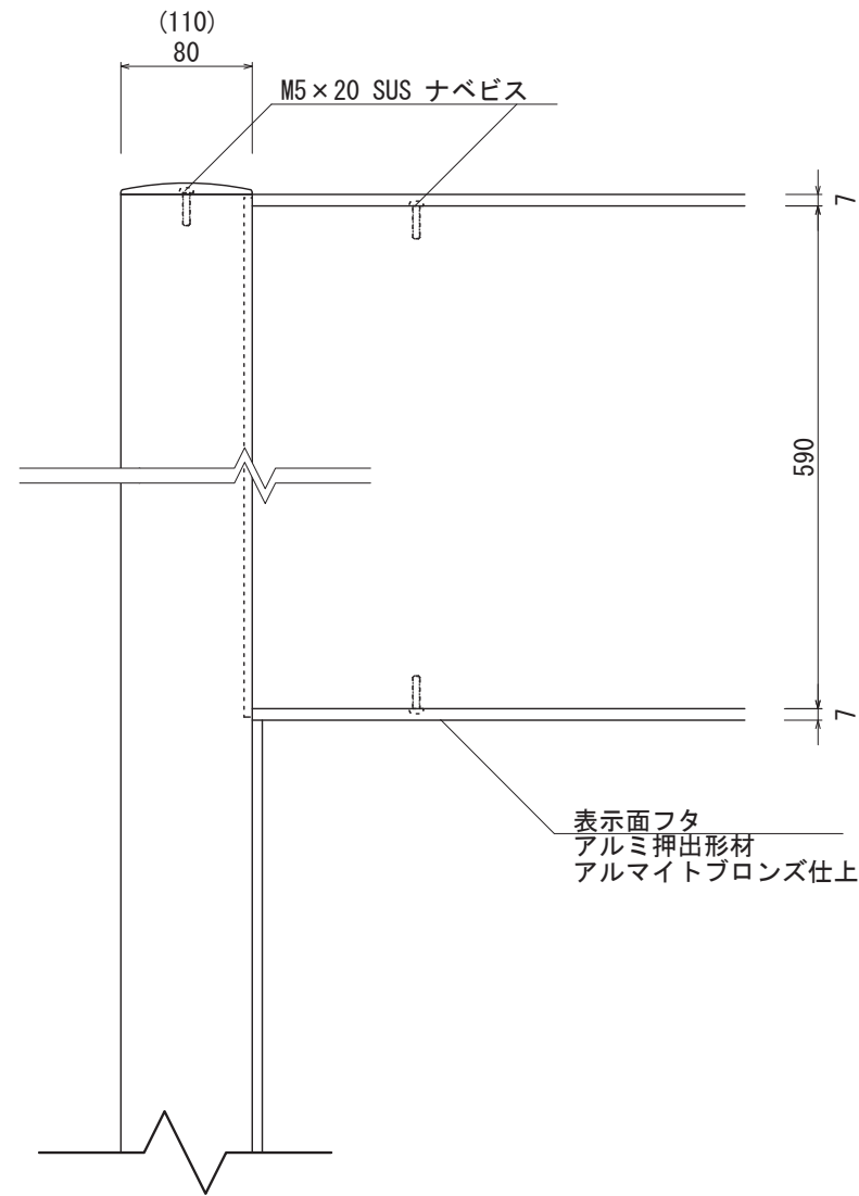
【正面図 S=1:5】
