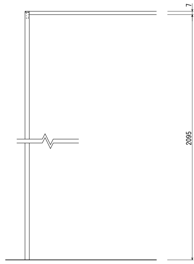
【正面図 S=1:5】
