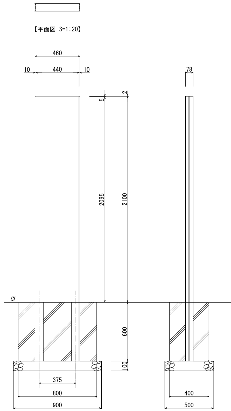
【正面図 S=1:20】
