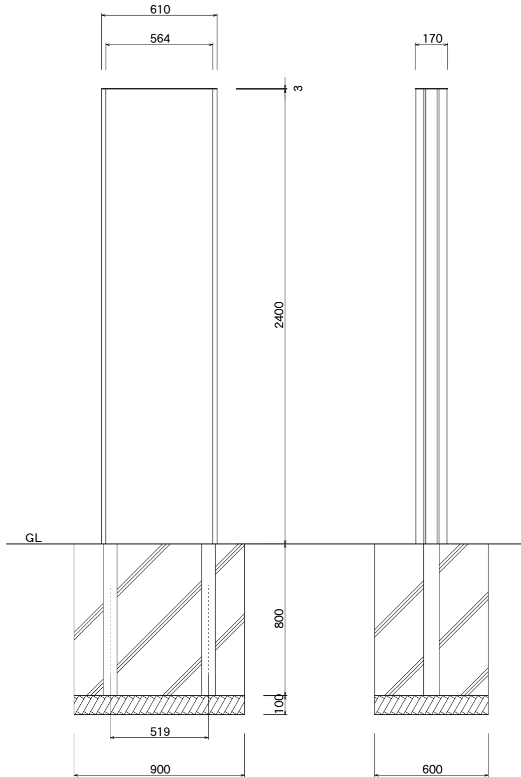
【正面図】
