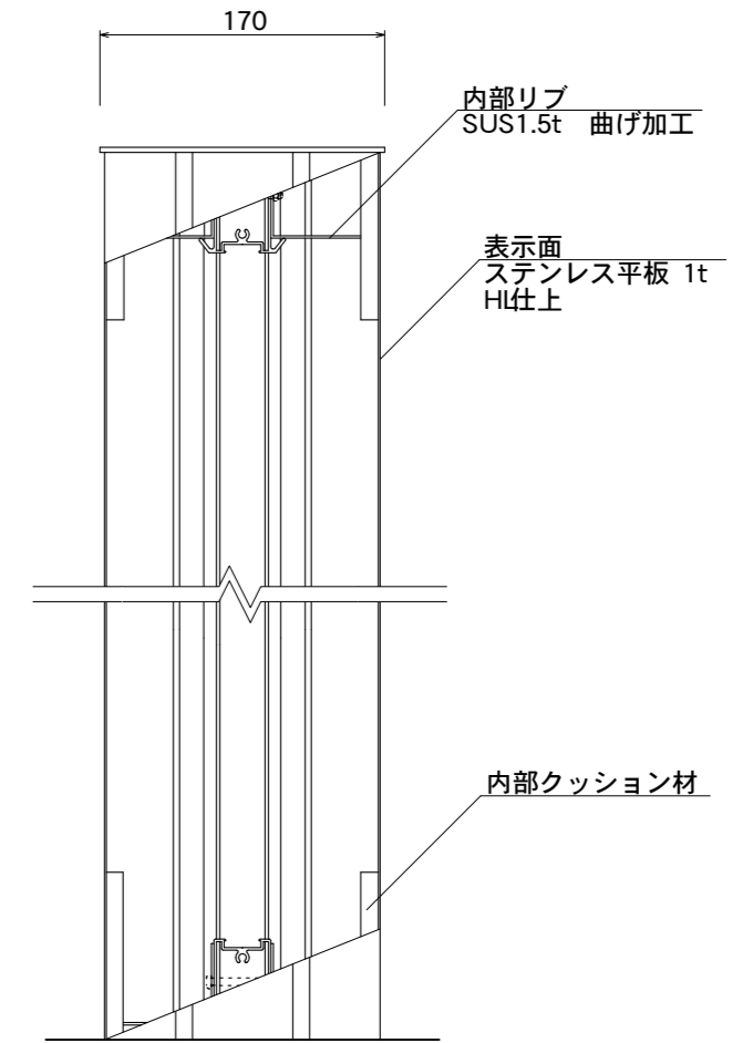
【側断面図】
