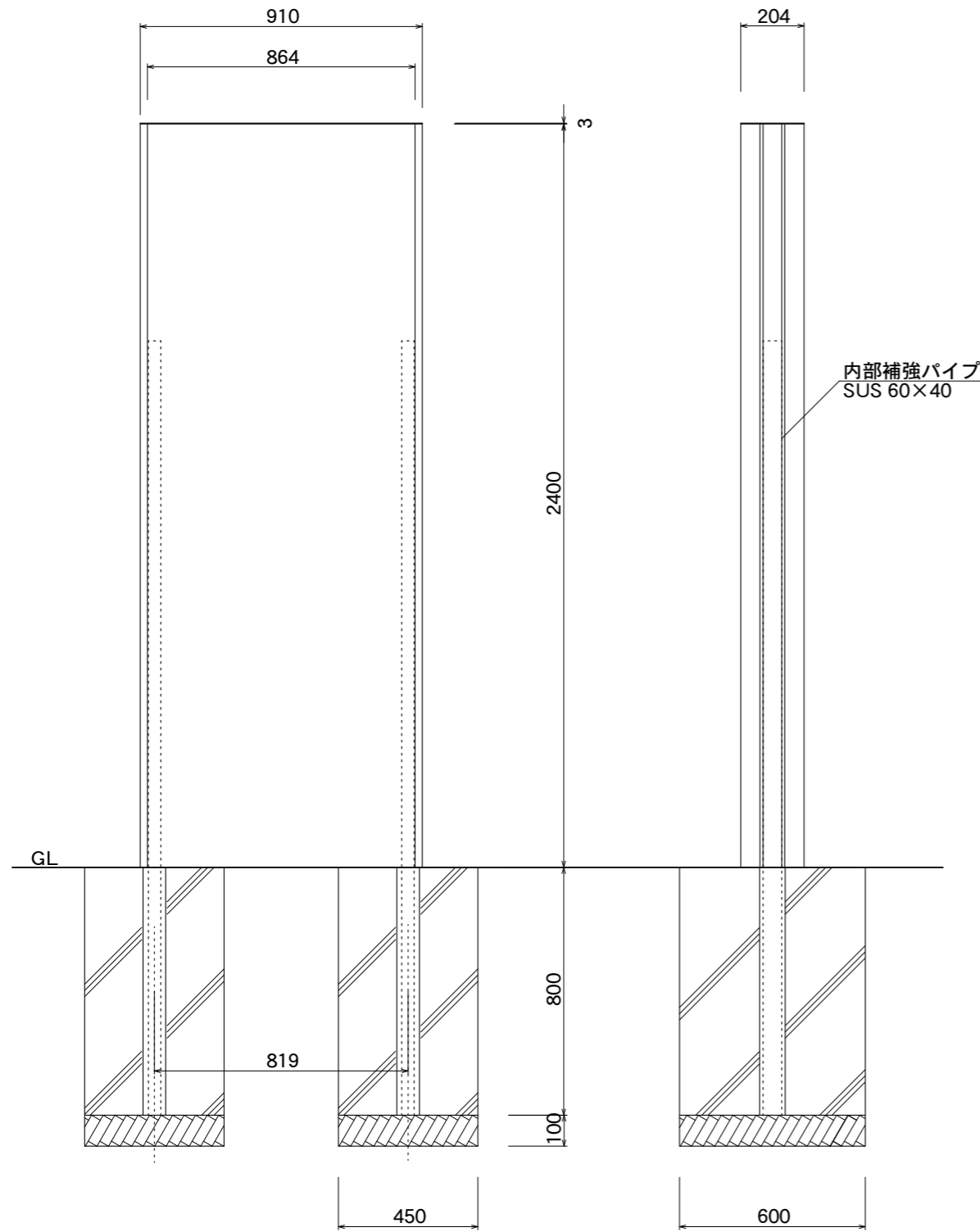
【正面図】
