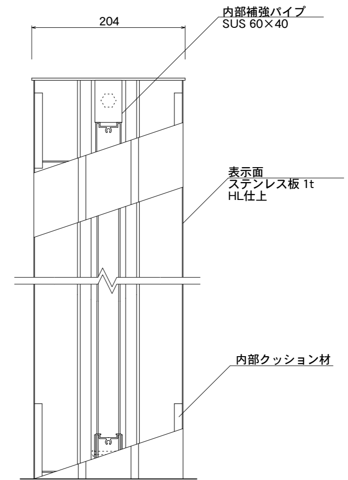
【側断面図】
